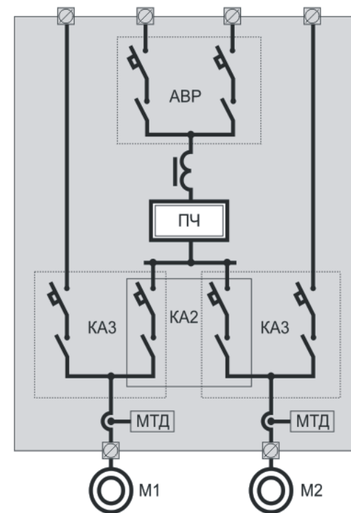
СТРУКТУРА СИЛОВЫХ ЦЕПЕЙ (схема для двух каналов)
